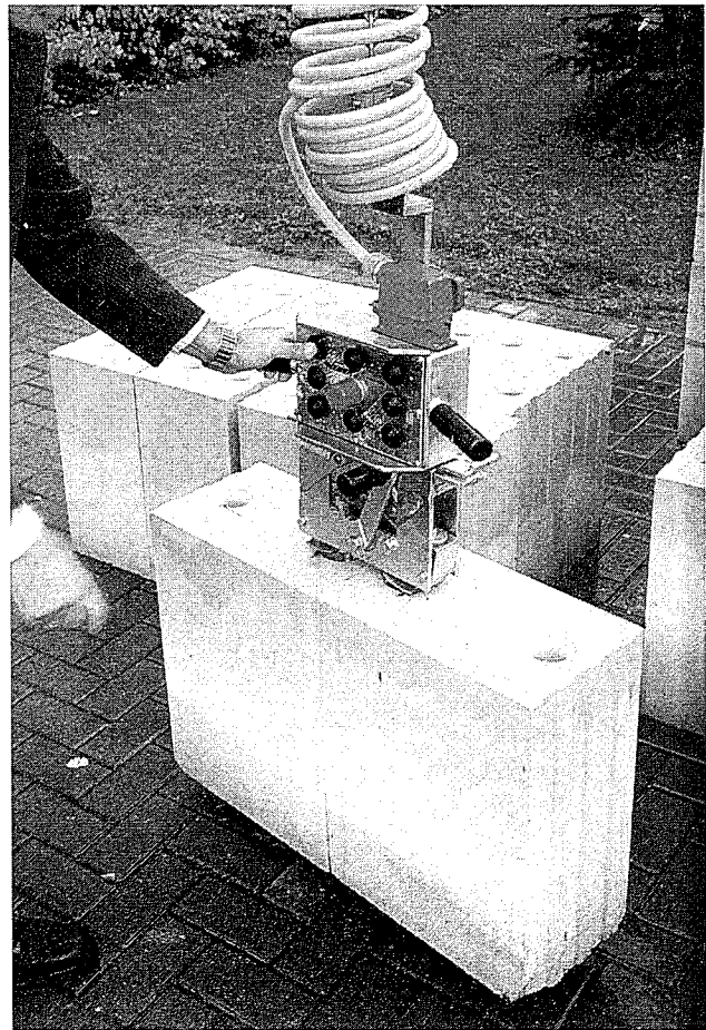
Quadroblokkkranens grip- och styrenhet
