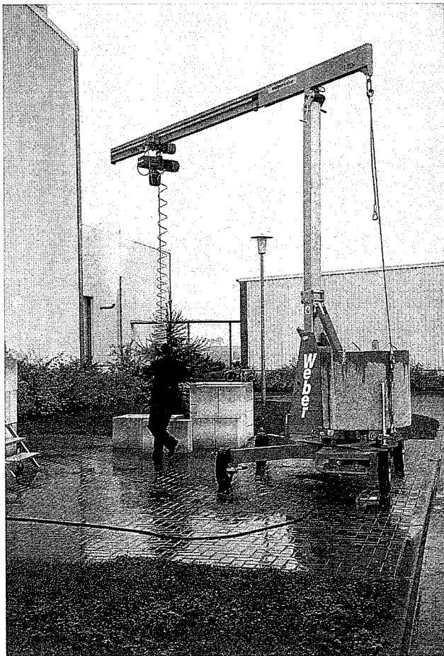
Muraren kan själv sköta och flytta kranen för Quadroblokk
