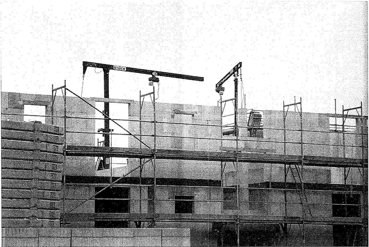
Quadroblokkmurning på två fronter
